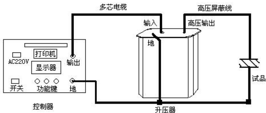
图 4 (连线图)
